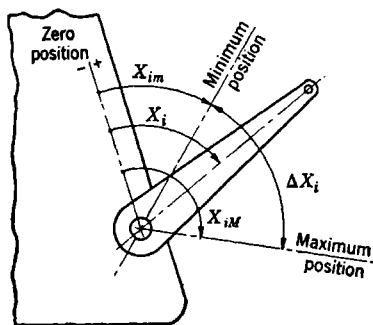
FIG. 3-1.—Crank terminal.
